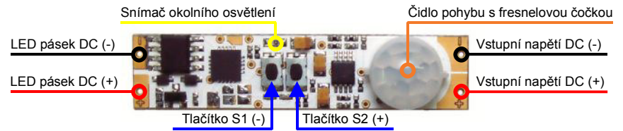
Obr.1 - Zapojení vývodů a umístění ovládacích prvků
